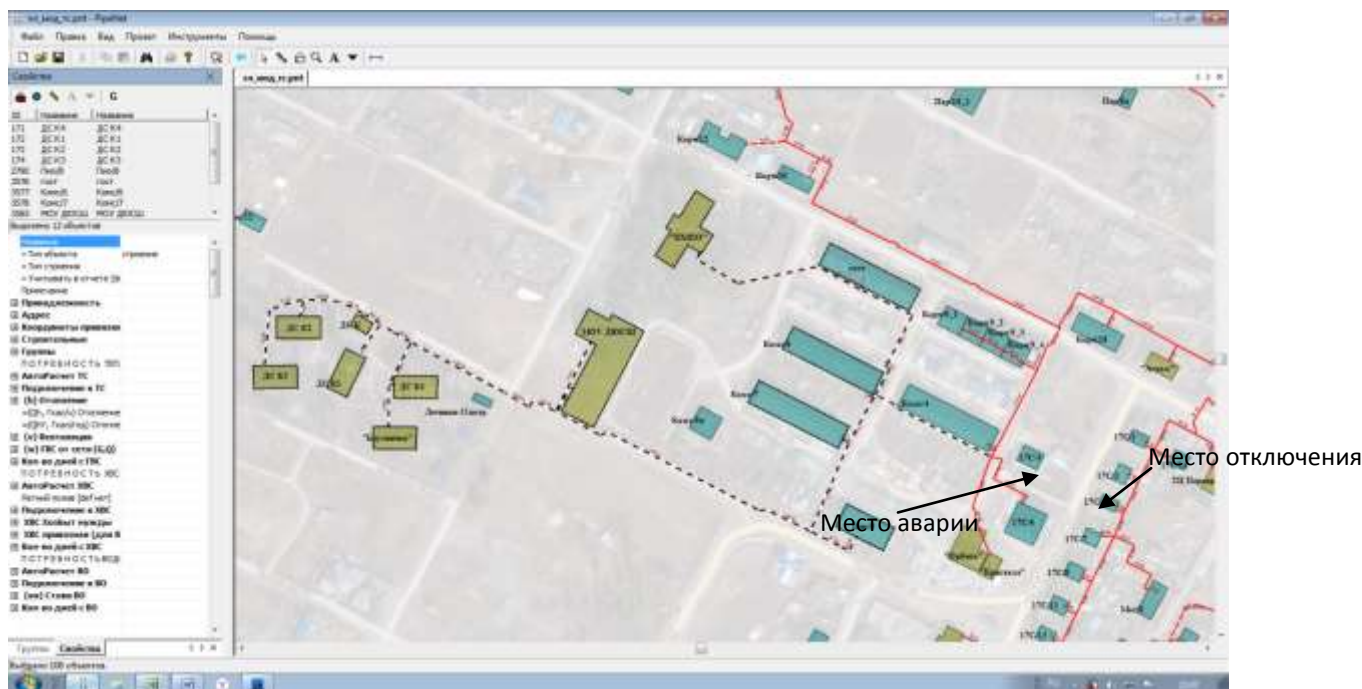
Рис. 2. Общий скрин электронной модели аварийной ситуации п. Магистральный. (пунктиром выделены объекты отключаемого района теплоснабжения)
