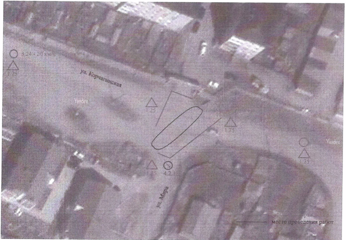
СХЕМА ОРГАНИЗАЦИИ ДОРОЖНОГО ДВИЖЕНИЯ и ограждения места производства работ по ул. Корчагинская в р.п. Магистральнинский
